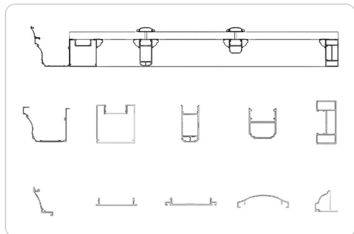
Чертежи профилей из каталога производителя, лист 23
